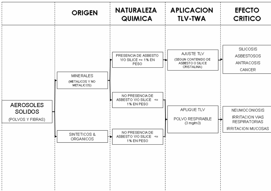
Figura 2. Proceso para determinar cuál TLV aplica según el origen, la naturaleza química y la presencia de sílice y/o asbestos en aerosoles sólidos.
