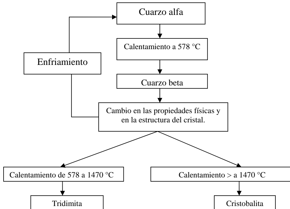
Figura 1 Influencia de la temperatura sobre la estructura cristalina del cuarzo (Castranova V et al, 2000).
